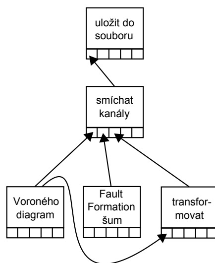
Obrázek 4.3: příklad grafového popisu
